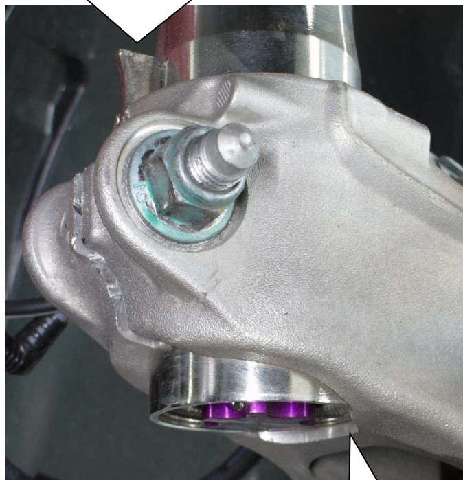
Anschlag / stop
