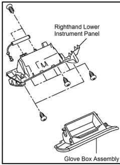
Fig. 1 Retrait du panneau d'instrument du bas. Nissan 370Z 2010-13
