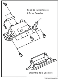
Fig. 1 Retiro del panel de instrumentos inferior. Nissan 370Z 2010-13
