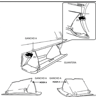
Fig. 1 Retiro de la guantera (Parte 1 de 3). Mazda CX-5 2013
