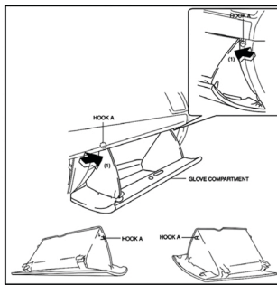
Fig. 1 Retrait du compartiment à gants (Part. 1 de 3). Mazda CX-5 2013
