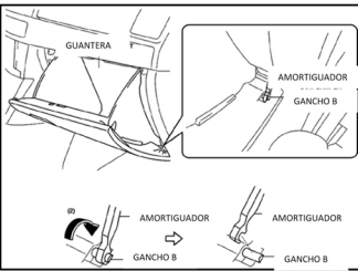
Fig. 1 Retiro de la guantera (Parte 2 de 3). Mazda CX-5 2013
