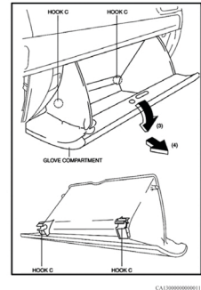
Fig. 1 Retrait du compartiment à gants (Part. 3 de 3). Mazda CX-5 2013
