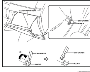
Fig. 1 Retrait du compartiment à gants (Part. 2 de 3). Mazda CX-5 2013
