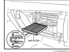
Fig. 2 Retrait du filtre à air de l'habitacle. Mazda CX-5 2013
