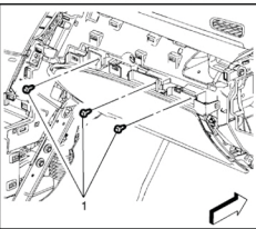
Fig. 5 Retiro de los sujetadores superiores del compartimento del panel de instrumentos. Cadillac XTS 2013.
