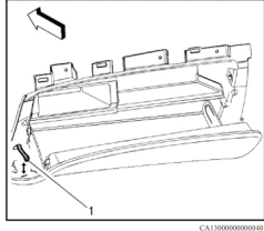
Fig. 6 Desconexión del amortiguador de la puerta del compartimento del panel de instrumentos. Cadillac XTS 2013.
