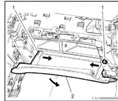
Fig. 7 Arrêts de porte du compartiment du panneau d'instruments. Cadillac XTS 2013
