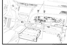
Fig. 9 Retiro del control de reproductor de discos de video. Cadillac XTS 2013.
