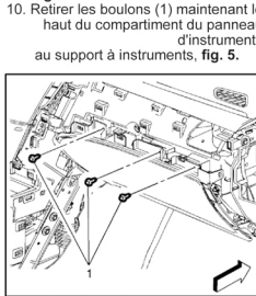
Fig. 5 Retrait de l'attache supérieure de la porte du compartiment du panneau d'instruments. Cadillac XTS 2013
