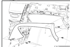
Fig. 4 Retrait de la garniture du panneau du bas. Cadillac XTS 2013
