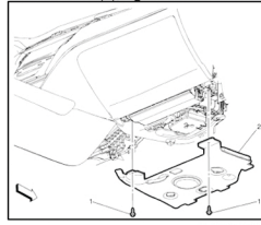
Fig. 1 Retrait du panneau d'isolation du panneau d'instruments de droite. Cadillac XTS 2013
