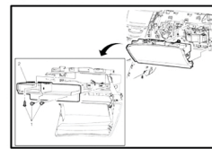
Fig. 10 Retiro de la bandeja del compartimento del panel de instrumentos. Cadillac XTS 2013.
