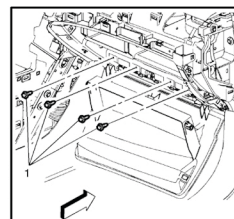
Fig. 8 Retrait de l'attache inférieure de la porte du compartiment du panneau d'instruments. Cadillac XTS 2013
