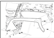
Fig. 4 Retiro del panel recortado inferior. Cadillac XTS 2013.
