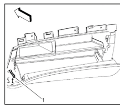
Fig. 6 Débranchement du vérin de la porte du compartiment du panneau d'instruments. Cadillac XTS 2013
