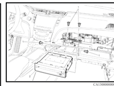
Fig. 9 Retrait du contrôle de lecteur de disque numérique. Cadillac XTS 2013
