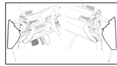
Fig. 2 Retrait du panneau du côté droit. Cadillac XTS 2013
