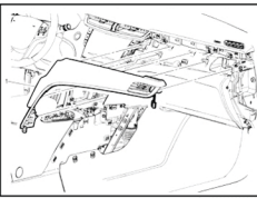
Fig. 3 Retiro del panel recortado superior. Cadillac XTS 2013
