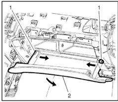
Fig. 7 Topes de la puerta del compartimento del panel de instrumentos. Cadillac XTS 2013
