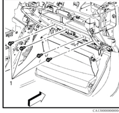
Fig. 8 Retiro de los sujetadores inferiores del compartimento del panel de instrumentos. Cadillac XTS 2013.
